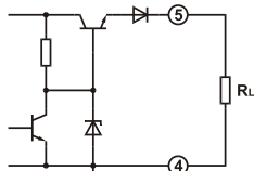
Abb. 4: Alarmausgang
