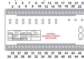
Abb. 1: Klemmen-Numerierung
