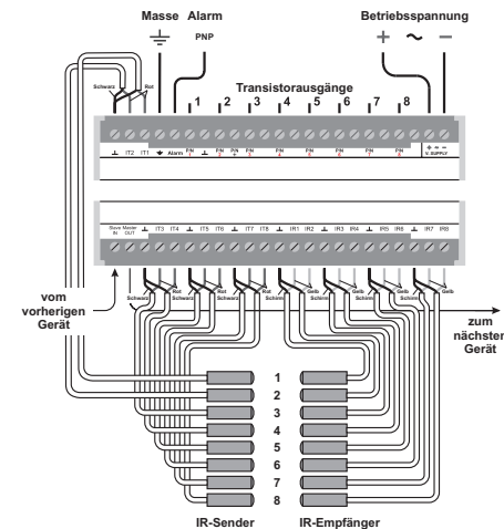
Abb. 2: Anschlussschema
