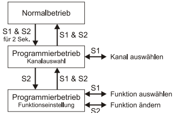
Abb. 6: Übersichtsbild Programmierbetrieb
