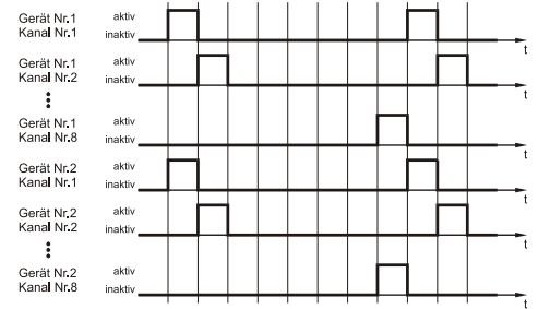
Abb. 7: Funktionsdiagramm Master-Slave-Betrieb
