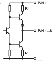
Abb. 3: Transistorausgang
