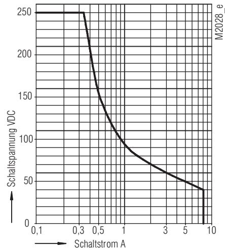
Lichtbogengrenzcurve
