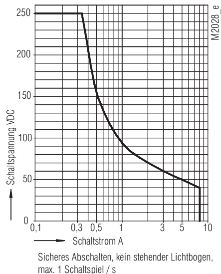
Lichtbogengrenzkurve
