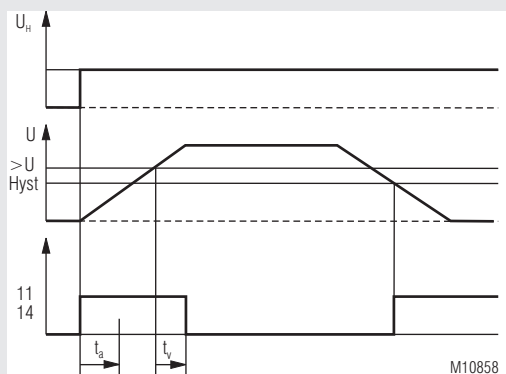
Beispiel: Überspannungsüberwachung mit Ruhestromprinzip
