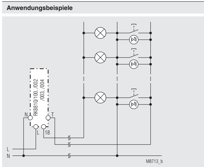
3-Leiter-Schaltung (N-getastet)
