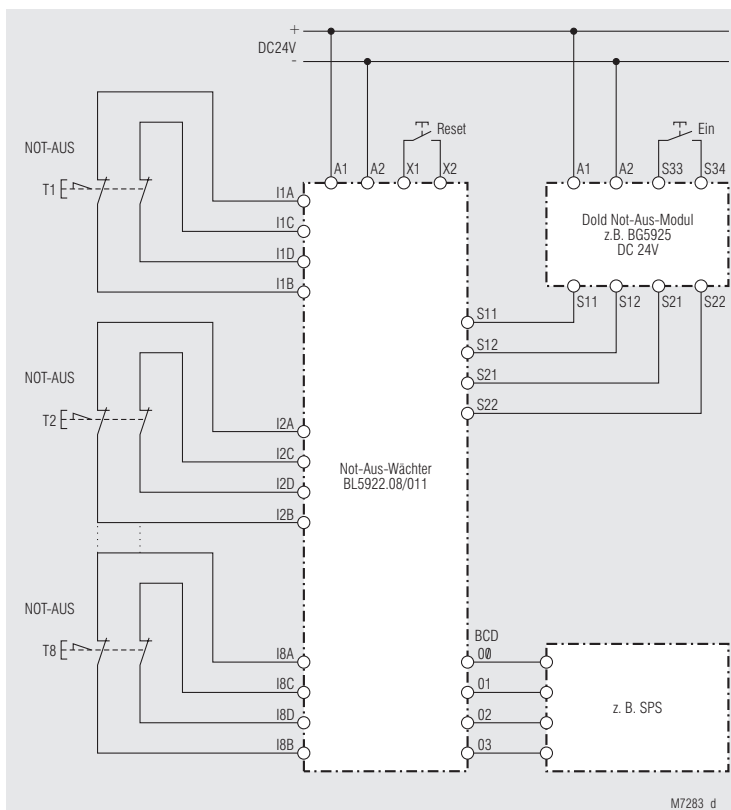
Bild 5: Überwachung von 8 Not-Aus-Tastern mit Not-Aus-Wächter, 2-kanaliger Anschluss, BCD-Ausgang, 1-kanalige Überwachung
