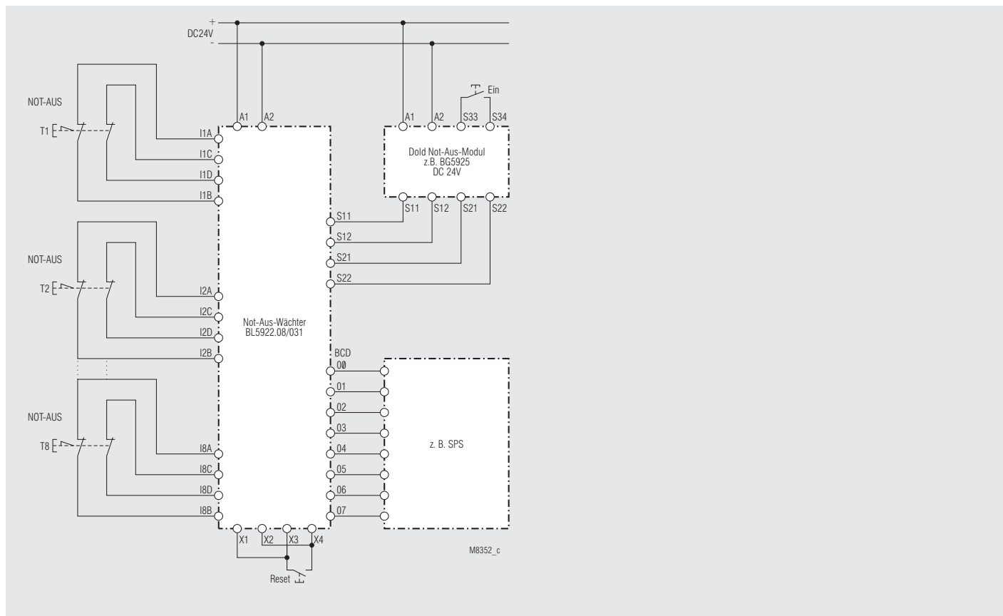
Bild 6: Überwachung von 8 Not-Aus-Tastern mit Not-Aus-Wächter, 2-kanalige Überwachung in querschlussssicheren Systemen, BCD-Ausgang.
