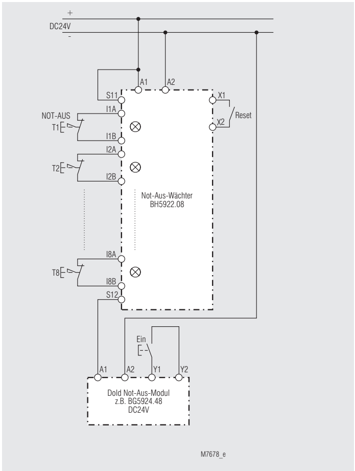
Bild 1: Überwachung von 8 Not-Aus-Tastern mit Not-Aus-Wächter, 1-kanaliger Anschluss, Not-Aus-Modul 1-kanalig. Anzeige über 8 frontseitige LEDs am Gerät.
