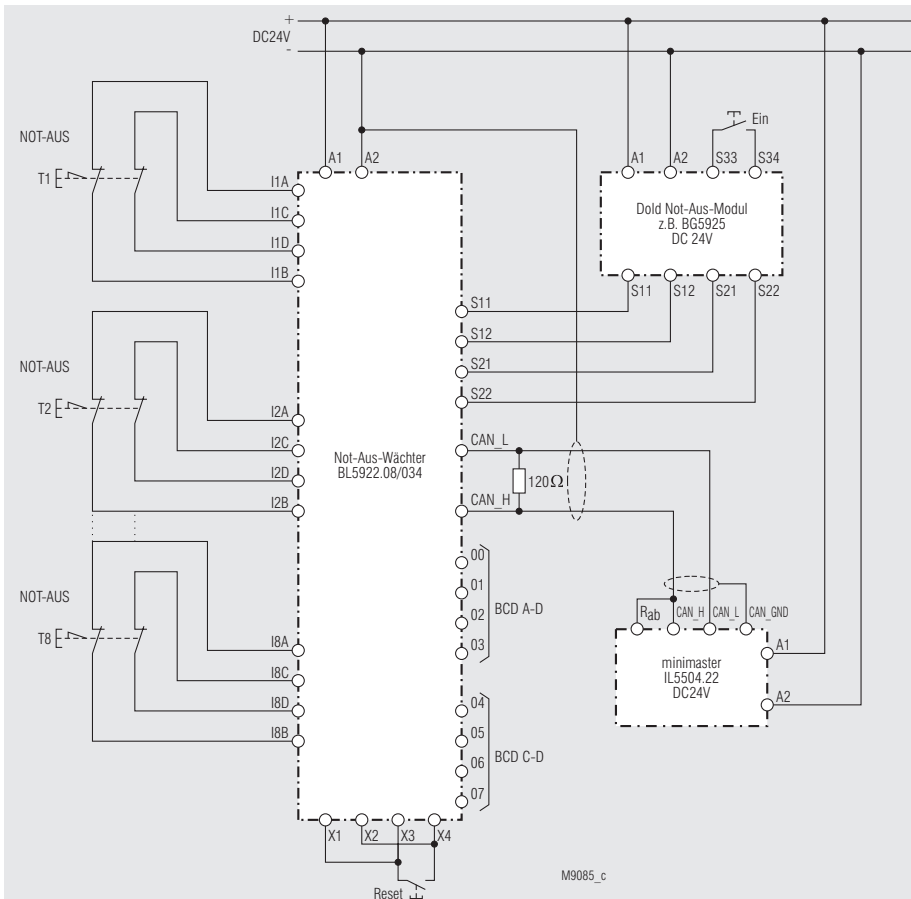
Bild 8: Überwachung von 8 Not-Aus-Tastern mit Not-Aus-Wächter, 2-kanaliger Anschluss, 2-kanalige Überwachung in querschluss sicheren Systemen mit CANopen minimaster IL 5504
