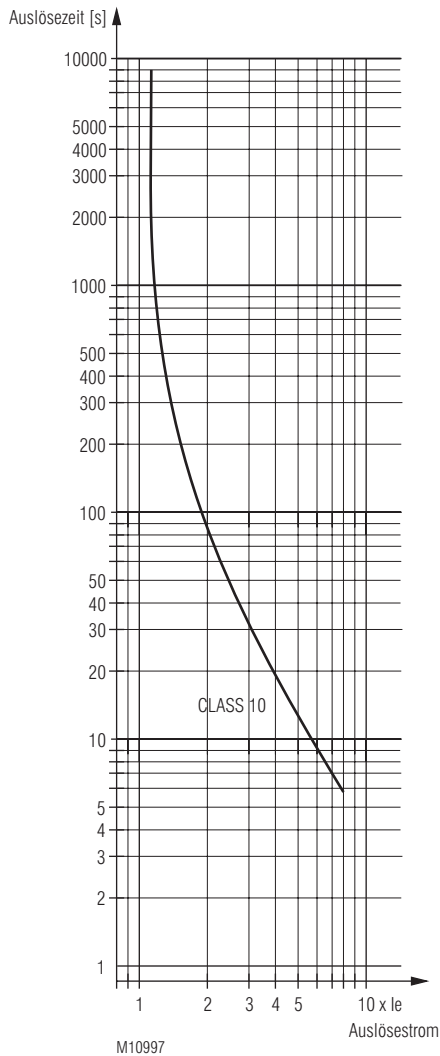
Auslösekennlinie
